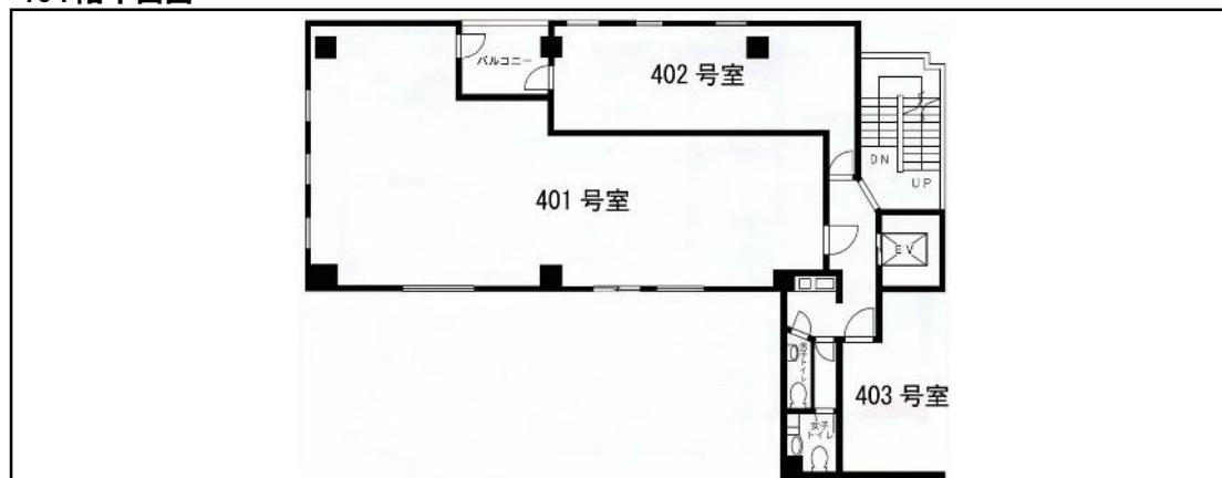
401階平面図
