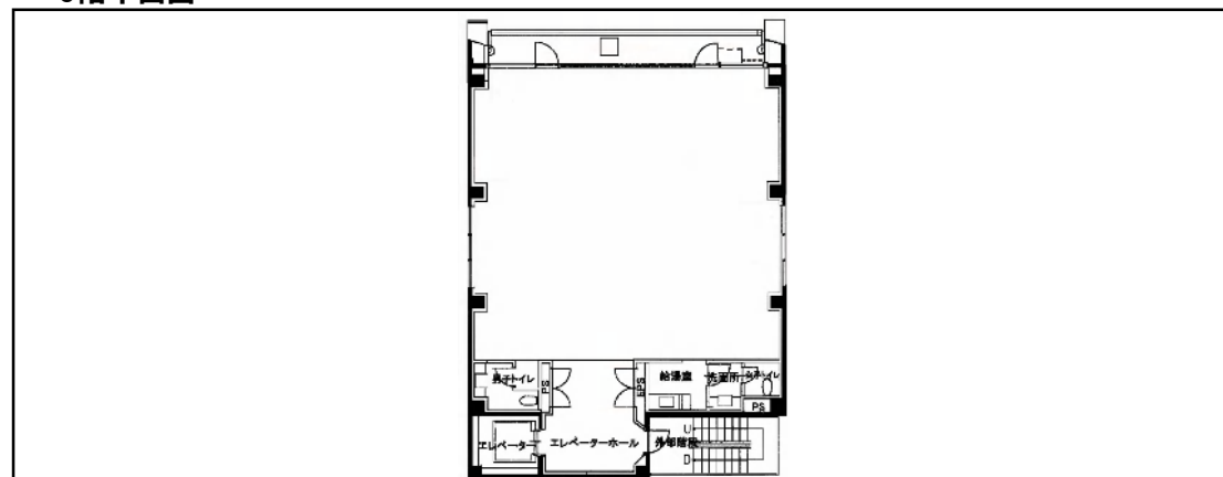
6階平面図
